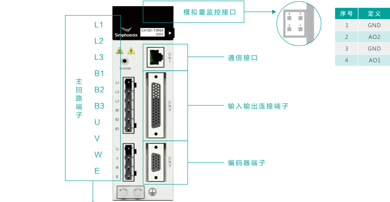
主回路端子的名称及功能
