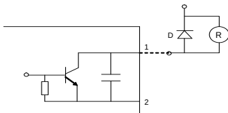
图 6-8 OC 输出端子的内部线路
