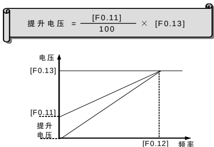
图 6-4 转矩提升示意图
