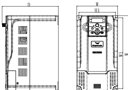
图 2-2-C 变频器安装尺寸 3
