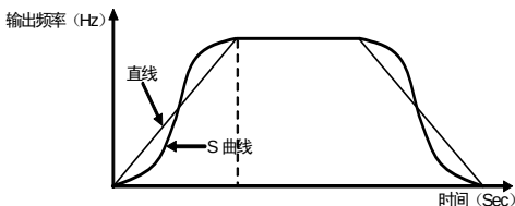
图 6-3 加减速曲线
