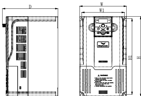
图 2-2-D 变频器安装尺寸 4
