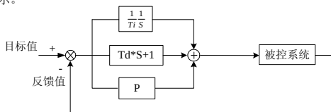
图 6-18 PID 作用示意图
