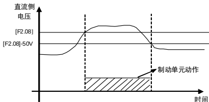
图 6-14 能耗制动
