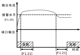
图 6-11 过载报警
