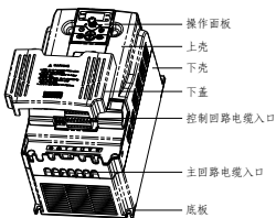
图 1-5 V类变频器外观及部件名称
