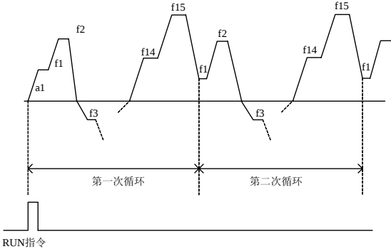
图 7-47-D 简易 PLC 运行连续循环模式
