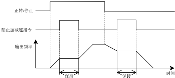
图 7-32 禁止加减速示意图
