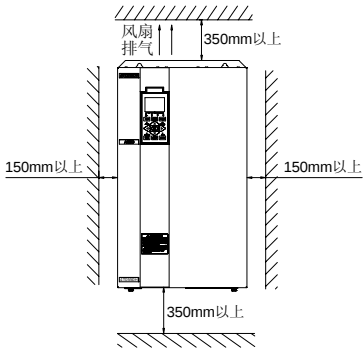
图 3-1-B 安装的间隔距离(15KW 以上)
