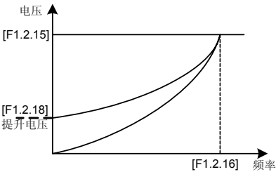
图 7-26-A 降转矩曲线转矩提升示意图
