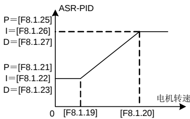
图 7-62-B 双 PID 参数（连续切换）
