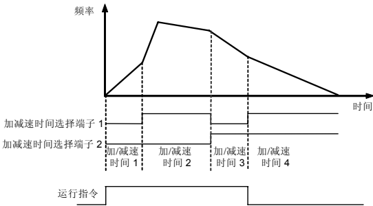
图 7-24 加、减速时间的外部端子选择方式
