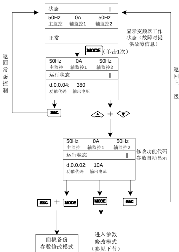
图 5-1 状态参数查询示意图
