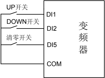
图 7-11 端子 UP/DW 接线示意图
