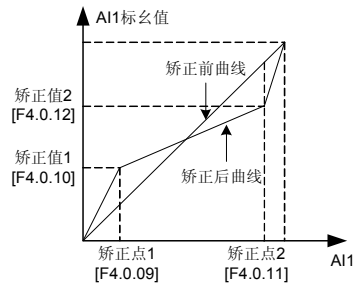
图 7-37 模拟输入 AI1 曲线矫正
