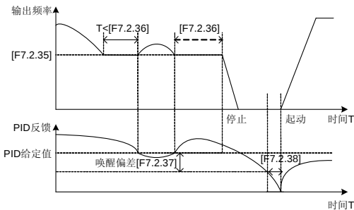
图 7-58 PID 睡眠功能示意图
