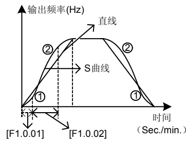
图 7-23 加减速曲线
