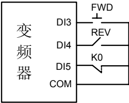
图 7-13-B 三线式运行模式 2
