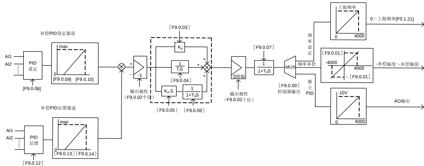
图 7-63 补偿 PID 原理框图
