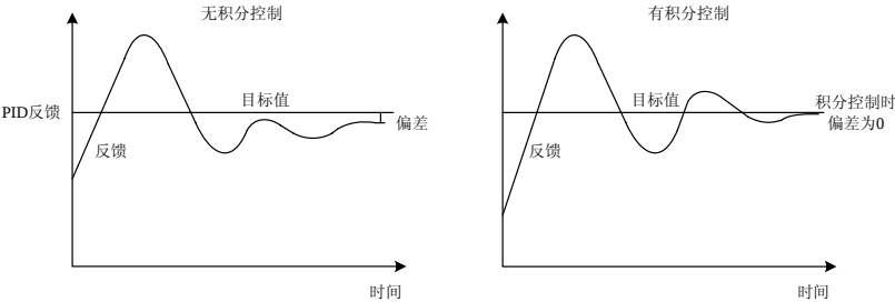
图 7-53 积分控制的作用
