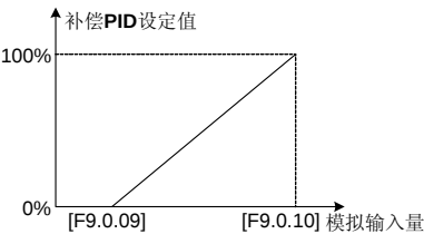
图 7-64 补偿 PID 设定值定义示意图
