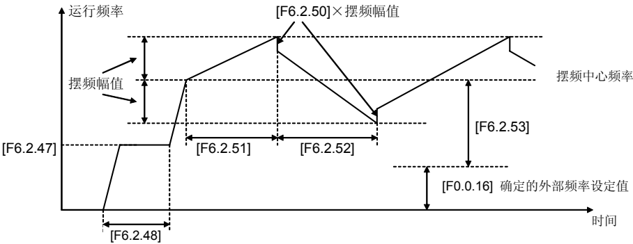
图 7-49 摆频运行示意图
