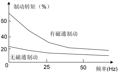
图 7-42 磁通制动曲线
