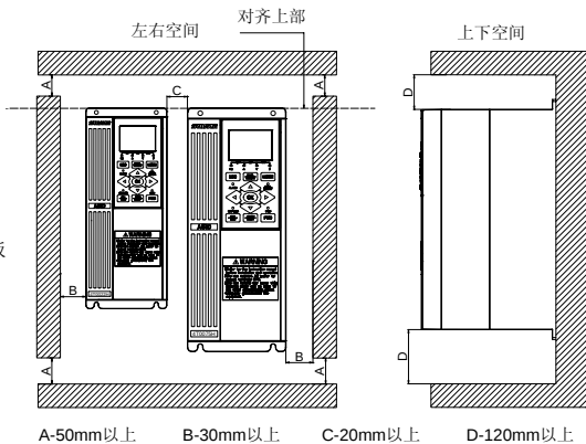
图 3-3 两台变频器（4.0KW 以上）左右安装尺寸
