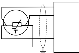
图 7-46-C 电机温度测量接线图 3
