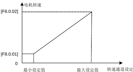
图 7-60 转速设定值和电机转速对应关系图
