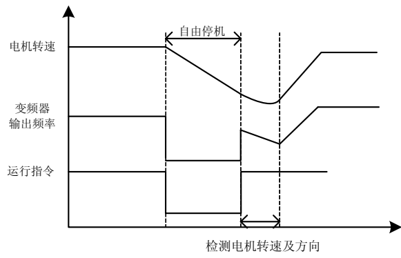
图 7-15 转速跟踪启动示意图
