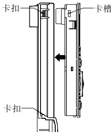
图 3-6 操作面板安装示意图
