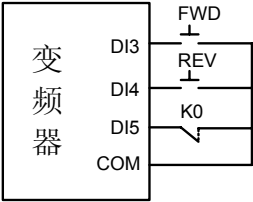
图 7-13-A 三线式运行模式 1
