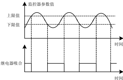
图 7-33-A 监控器功能示意图 1
