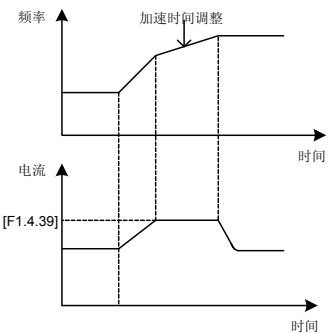
图 7-29 加/减速电流限制示意图
