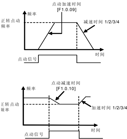
图 7-10 正转点动运行曲线
