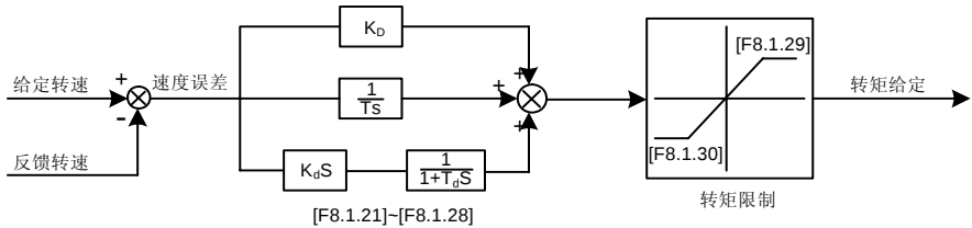
图 7-59 转速闭环框图
