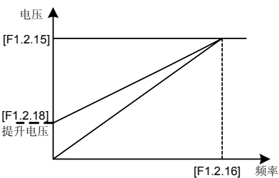
图 7-26-B 恒转矩曲线转矩提升示意图
