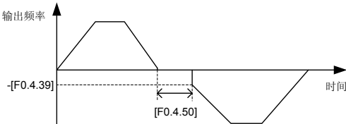
图 7-21 启动频率正反转切换示意图
