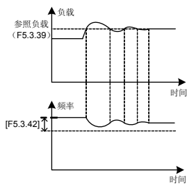
图 7-44 负载动平衡功能示意图
