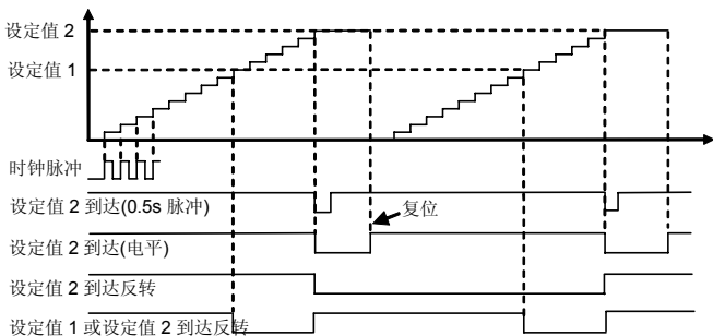
图 7-41-B 计数器功能 2
