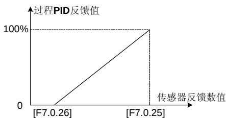
图 7-57 反馈百分比与对应传感器数值的关系曲线
