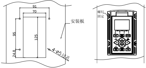
图 3-10-B 操作面板安装尺寸 2
