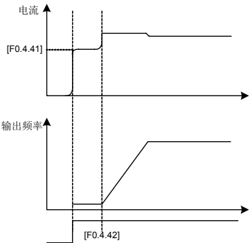
图 7-17 启动预励磁输出
