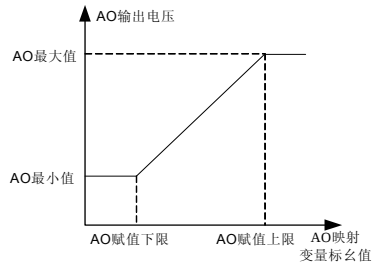
图 7-38 AO 输出特性曲线
