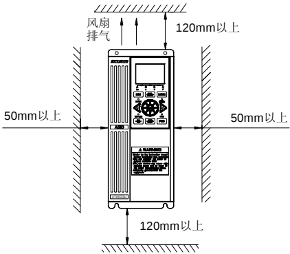
图 3-1-A 安装的间隔距离(11KW 及以下)
