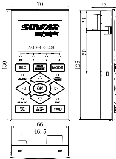
图 3-10-A 操作面板安装尺寸 1
