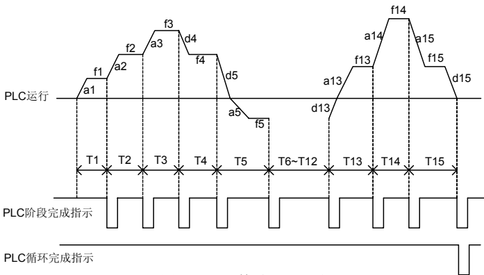
图 7-47-A 简易 PLC 运行
