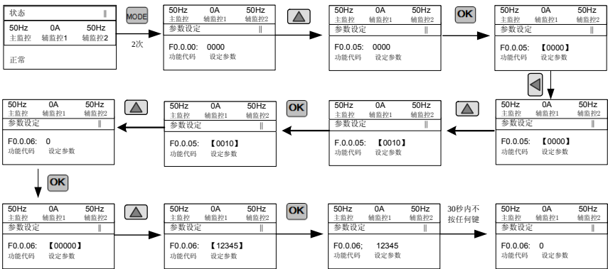
图 7-4 参数锁定操作流程
