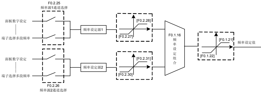
图 7-7 频率设定通道结构示意图
