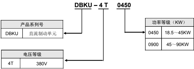
图 12-1 型号说明示意图
