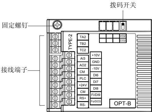
图 12-8 I/O 扩展卡示意图
