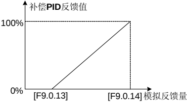
图 7-65 补偿 PID 反馈值定义示意图
