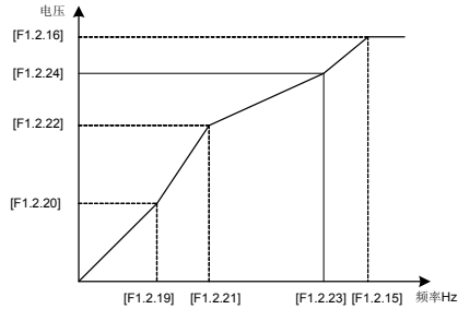
图 7-27 V/F 自定义曲线
