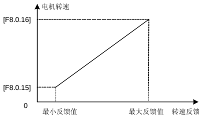
图 7-61 转速反馈值和电机转速对应关系图
