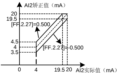
图 7-69-A AI2 零偏矫正曲线
