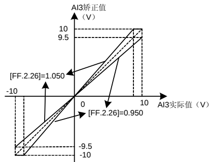
图 7-70-B AI3 增益矫正曲线
