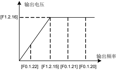
图 7-9 频率参数定义示意图
