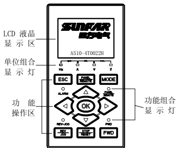
图 3-4-A LCD 标准型
