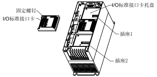
图 12-6 I/O 标准接口卡的拆卸安装示意图
