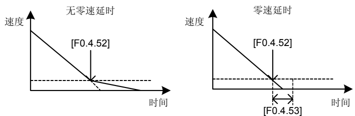
图 7-22 有无零速延时对比图
