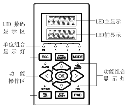
图 12-10-A LED 按键型
