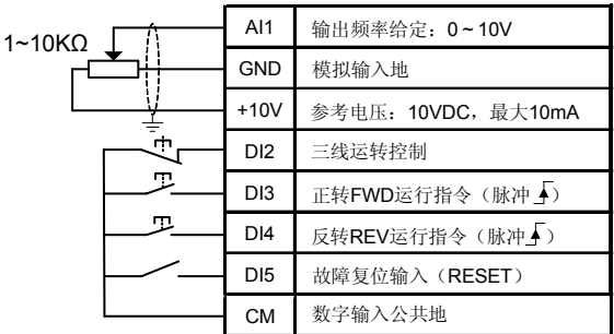
图 7-3 三线控制一 / AI1 设定接线图
