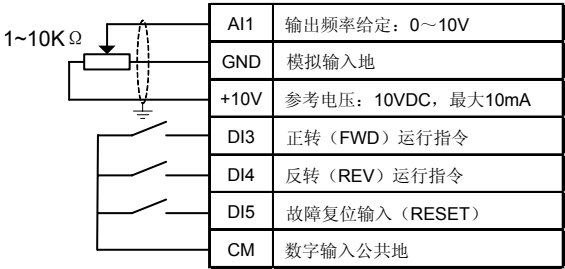
图 7-2-A 两线控制一/AI1 设定接线图
