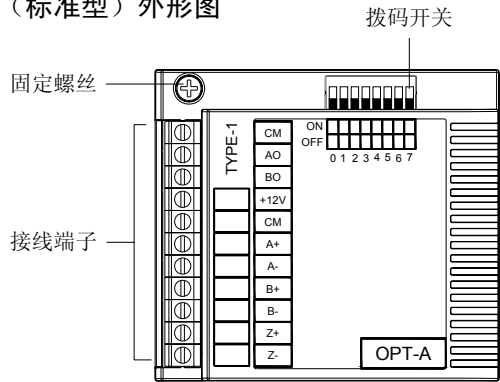
图 12-9 PG 卡（标准型）示意图
