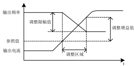
图 7-45 动平衡变量设置示意图
