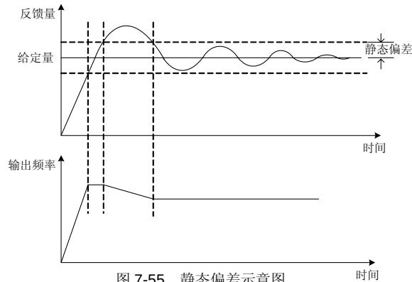
图 7-55 静态偏差示意图
