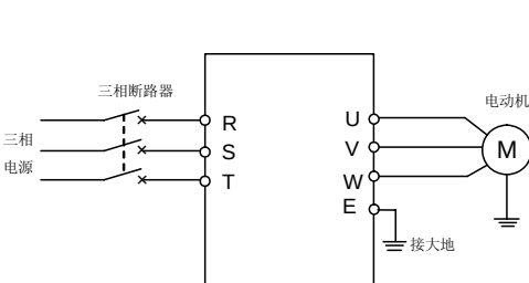
图 5-3 SVC 运行接线
