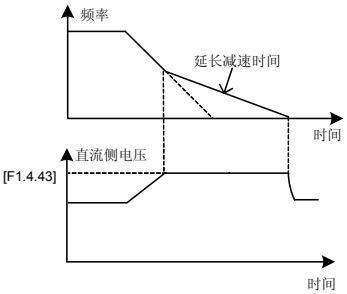
图 7-30-B 减速过程的过压抑制
