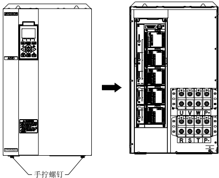
图 3-9 钣金盖板的拆卸安装示意图
