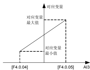
图 7-35-A AI1 模拟输入与对应变量示意图(单极性) 图 7-35-B AI3 模拟输入与对应变量示意图(双极性)
