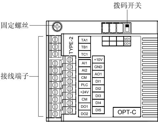
图 12-5 I/O 标准接口卡示意图
