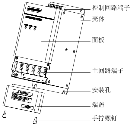
图 12-2 外观示意图
