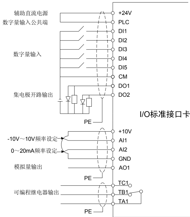
图 12-7 I/O 标准接口卡的配线图
