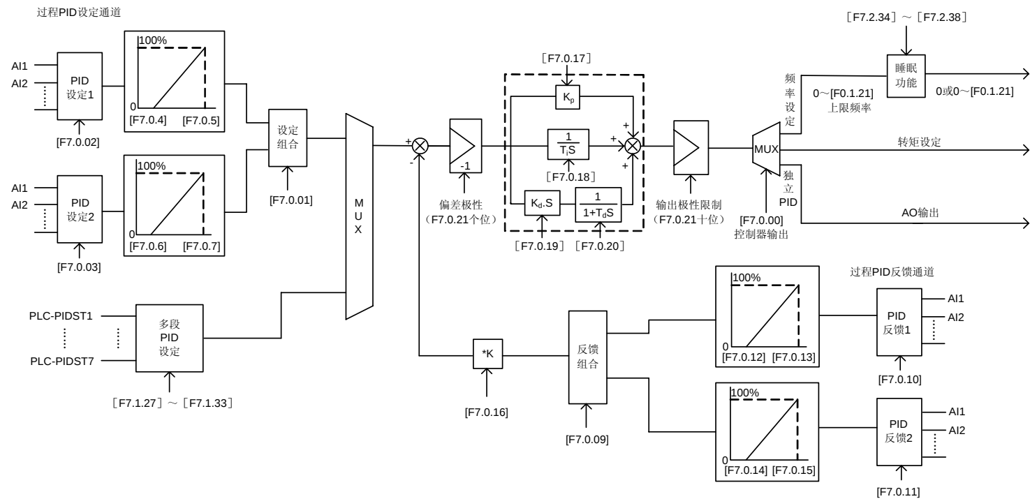
图 7-50 过程 PID 控制原理框图
