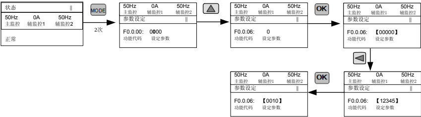
图 7-5 参数解锁操作流程
