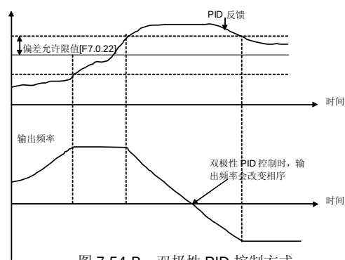
图 7-54-B 双极性 PID 控制方式
