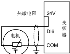
图 7-46-B 电机温度测量接线图 2
