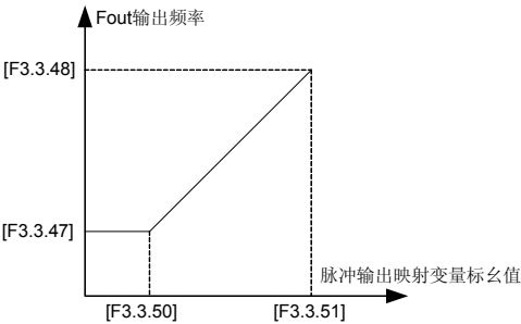
图 7-34 脉冲输出 Fout 特性曲线
