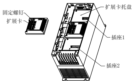
图 3-11 扩展卡的拆卸安装示意图
