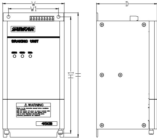
图 12-3 安装尺寸图
