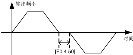
图 7-20 正反转过渡死区示意图
