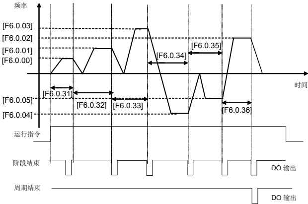
图 7-47-C 简易 PLC 运行单循环停机模式
