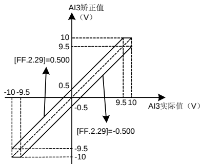
图 7-70-A AI3 零偏矫正曲线
