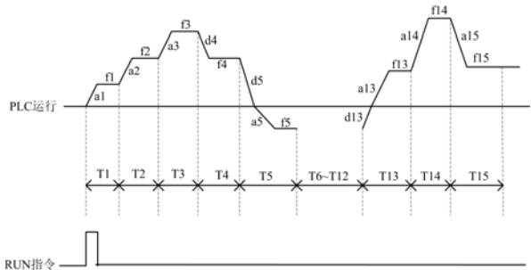
图 7-47-E 简易 PLC 运行保持最终值模式
