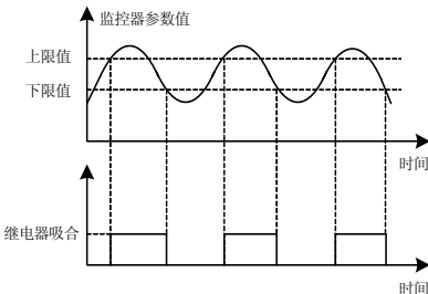
图 7-33-B 监控器功能示意图 2
