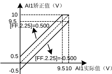
图 7-68-A AI1 零偏矫正曲线
