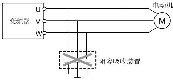
图 4-1 输出端禁止连接阻容吸收装置
