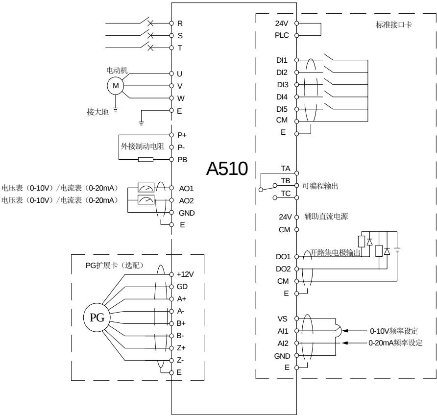
图 4-3 A510 系列变频器基本接线图
