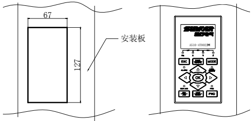
图 3-10-C 操作面板安装尺寸 3
