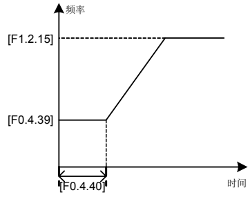
图 7-16 启动频率示意图
