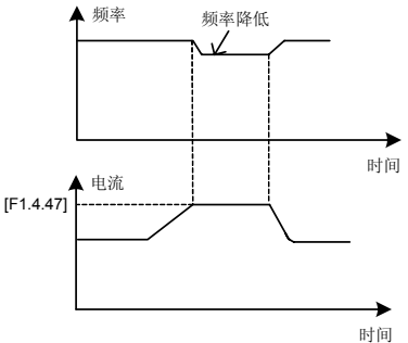
图 7-31-B 限流调节示意图
