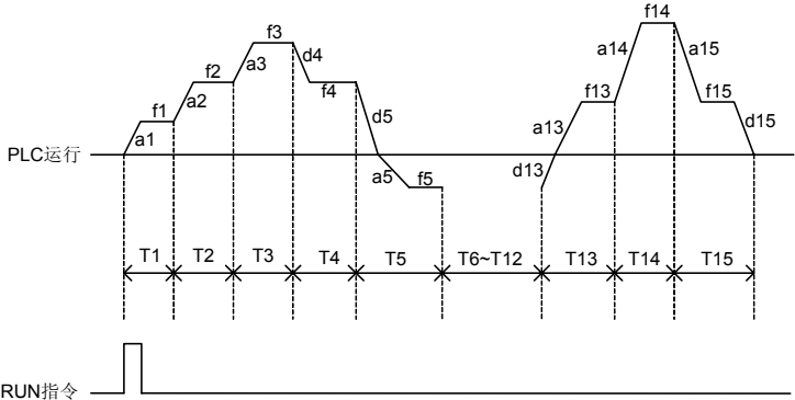
图 7-47-B 简易 PLC 运行单循环模式
