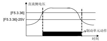
图 7-43 能耗制动
