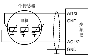
图 7-46-A 电机温度测量接线图 1
