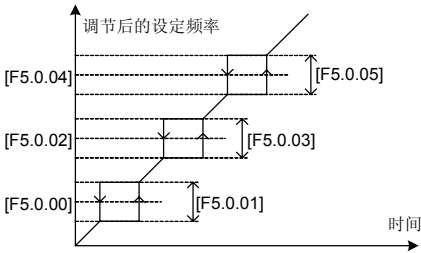
图 7-39 跳跃频率输出示意图
