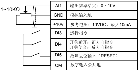
图 7-2-B 两线控制二 / AI1 设定接线图
