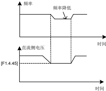
图 7-31-A 欠压调节示意图
