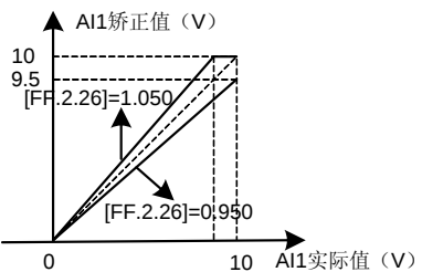
图 7-68-B AI1 增益矫正曲线
