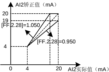
图 7-69-B AI2 增益矫正曲线
