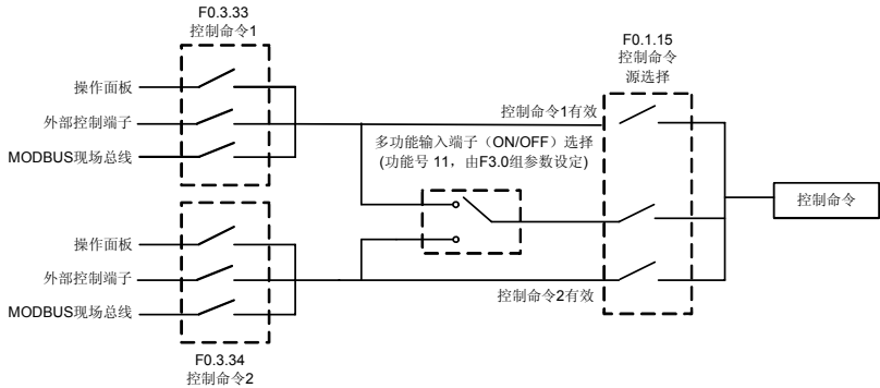
图 7-6 控制命令源选择示意图
