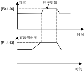
图 7-30-A 稳定运行过程的过压抑制
