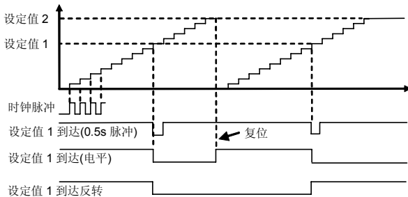
图 7-41-A 计数器功能 1
