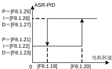
图 7-62-A 双 PID 参数（滞环切换）
