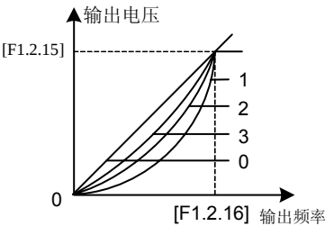
图 7-25 V/F 曲线
