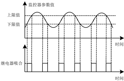
图 7-33-C 监控器功能示意图 3
