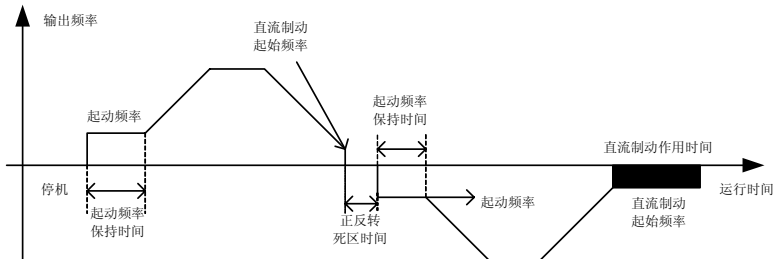
图 7-19 停机直流制动示意图
