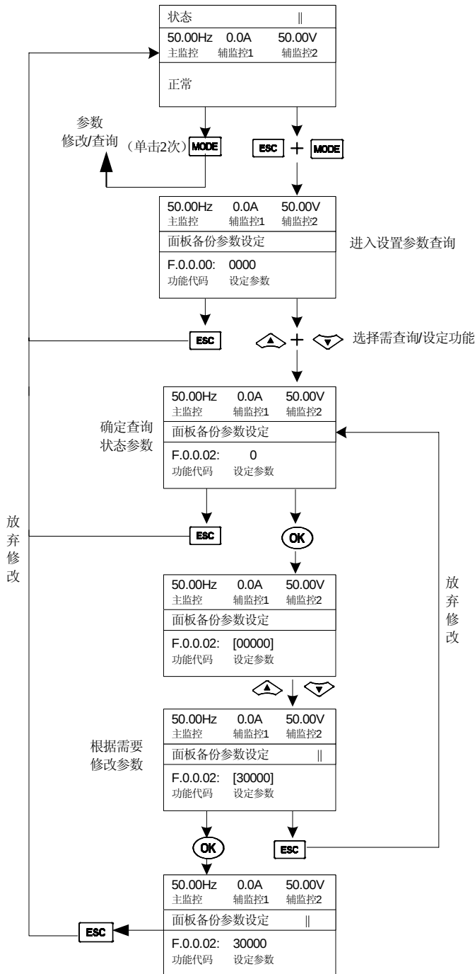
图 5-3 面板备份参数查询与修改示意图
