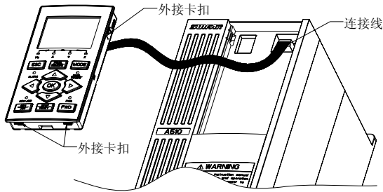
图 3-7 外延键盘连接线
