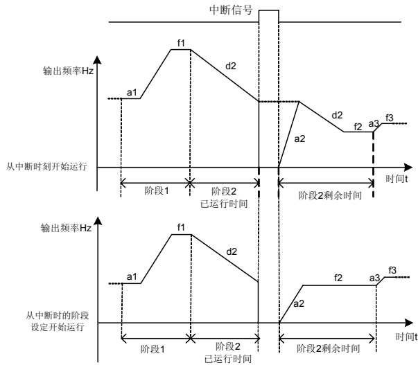
图 7-48 断点恢复示意图
