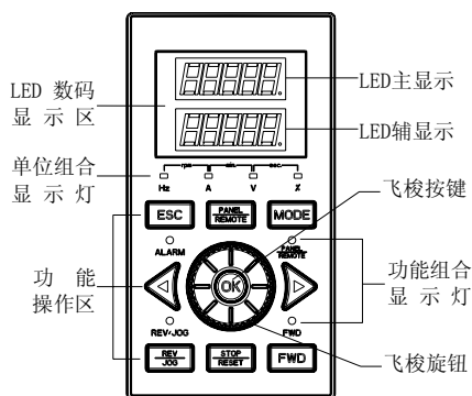
图 12-10-B LED 飞梭型
