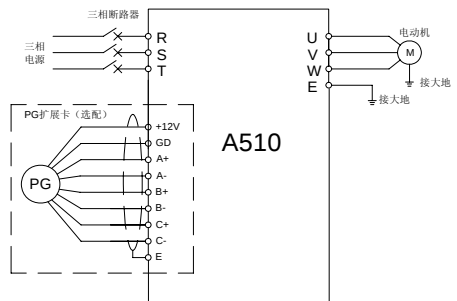
图 5-4 VC 运行接线图
