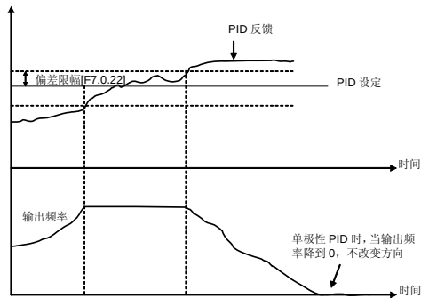
图 7-54-A 单极性 PID 控制方式
