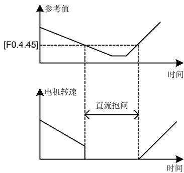
图 7-18 直流抱闸示意图
