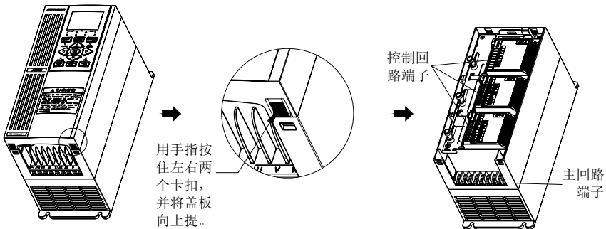
图 3-8 塑壳盖板的拆卸安装示意图
