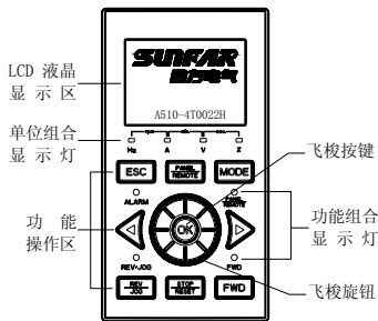
图 3-4-B LCD 飞梭型
