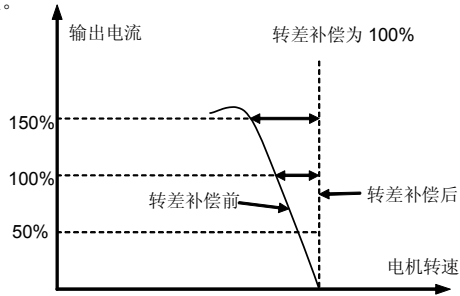
图 7-28 转差频率补偿示意图
