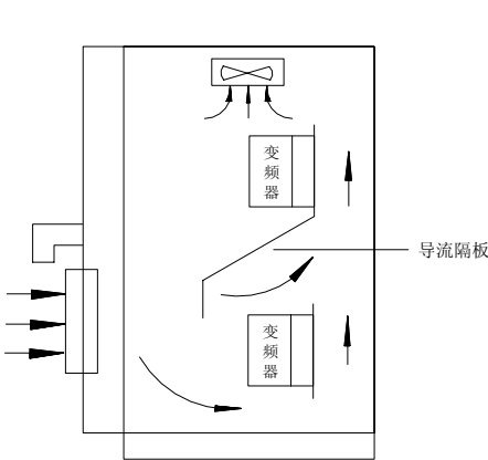
图 3-2 两台变频器上下安装间隔
