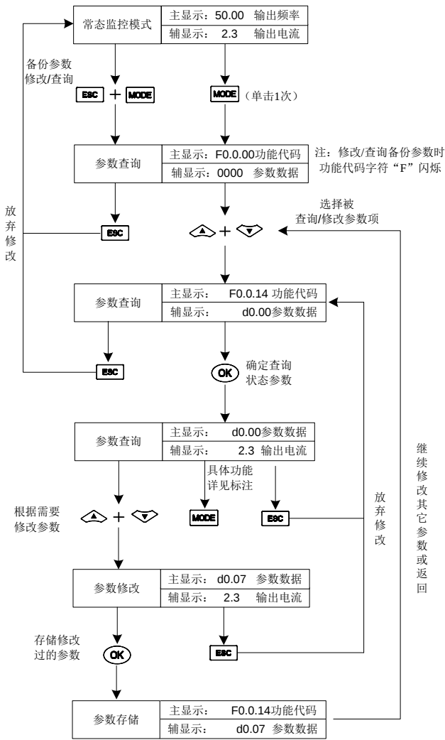
图 5-2 参数查询与修改示意图
