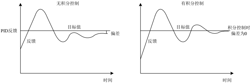
图 7-54 积分控制的作用
