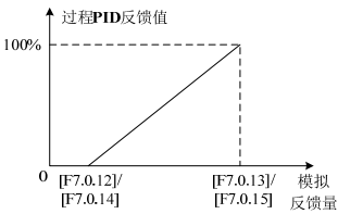
图 7-53 过程 PID 反馈值对应关系示意图
