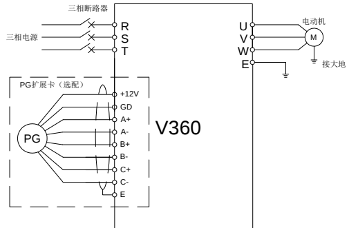
图 5-4 VC 模式运行接线
