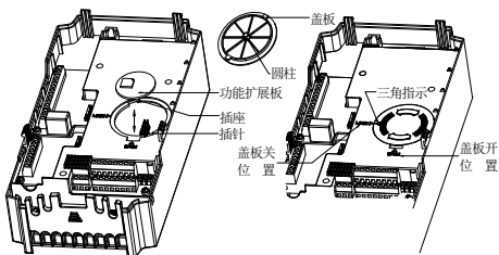
图 3-12 功能板的安装拆卸示意图
