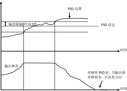
图 7-55-A 单极性 PID 控制方式
