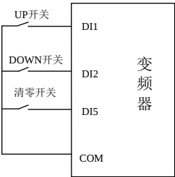
图 7-12 端子 UP/DW 接线示意图
