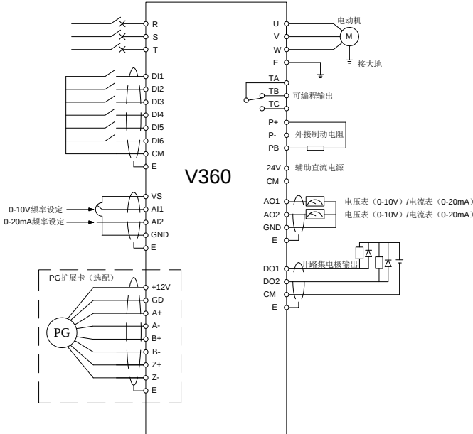
图 4-3 V360 系列变频器基本接线图
