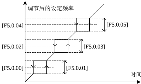
图 7-40 跳跃频率输出示意图
