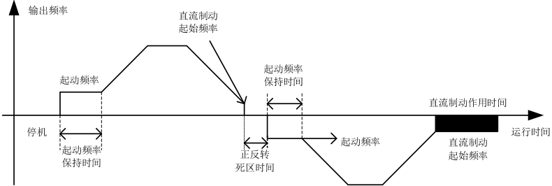
图 7-20 停机直流制动示意图
