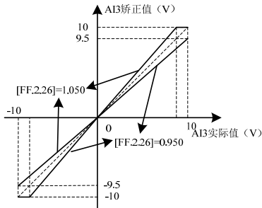
图 7-71-B AI3 增益矫正曲线
