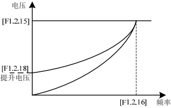
图 7-27-A 降转矩曲线转矩提升示意图
