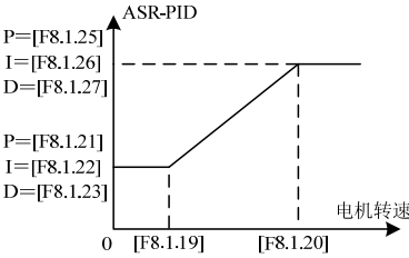
图 7-63-B 双 PID 参数（连续切换）
