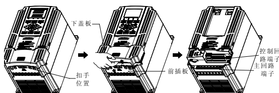
图 3-8 塑壳盖板的拆卸安装示意图
