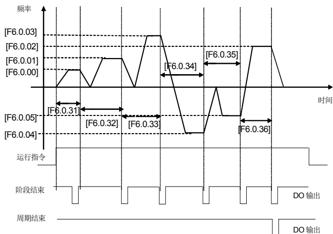
图 7-48-C 简易 PLC 运行单循环停机模式
