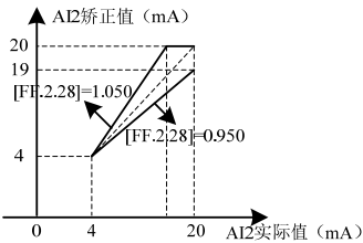
图 7-70-B AI2 增益矫正曲线
