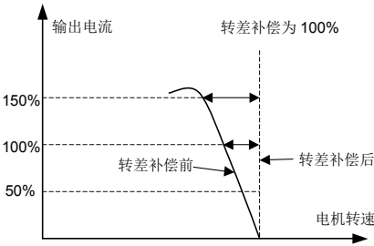
图 7-29 转差频率补偿示意图
