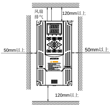
图 3-1-A 安装的间隔距离(45KW 及以下)
