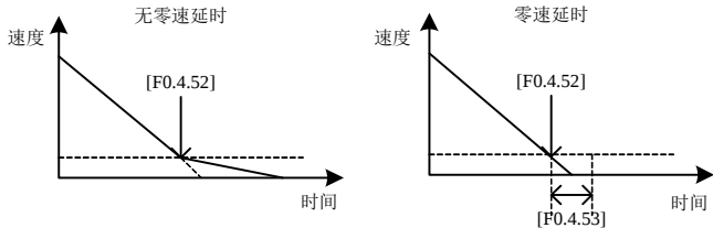
图 7-23 有无零速延时对比图
