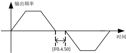
图 7-21 正反转过渡死区示意图
