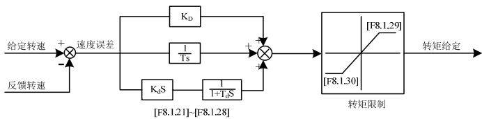
图 7-60 转速闭环框图
