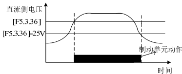
图 7-44 能耗制动
