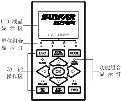
图 12-7-A 双语 LCD 标准型 (型号 DPNL360CA /PN: 050M007360001)
