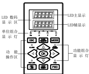
图 3-4-A 双 LED 标准型
