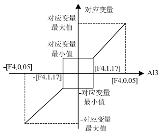
图 7-37-B AI3 模拟输入与对应变量示意图(双极性)
