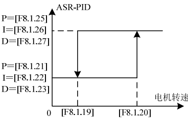
图 7-63-A 双 PID 参数（滞环切换）
