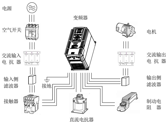
图 4-2 变频器的配线
