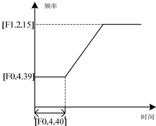
图 7-17 启动频率示意图
