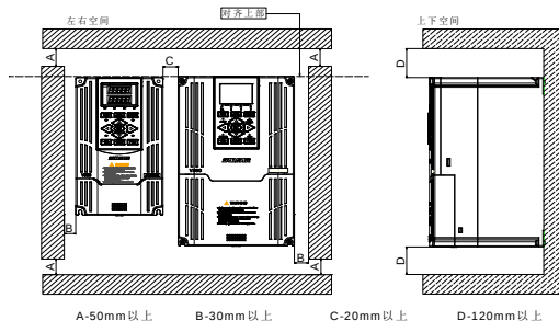
图 3-3 两台变频器（4.0KW 以上）左右安装尺寸
