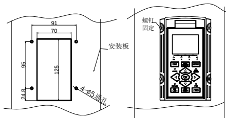
图 3-10-B 操作面板安装尺寸 2
