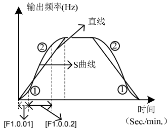
图 7-24 加减速曲线
