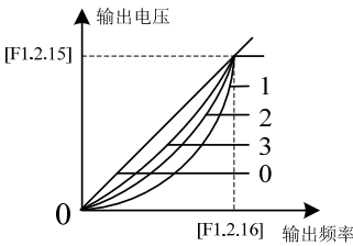
图 7-26 V/F 曲线
