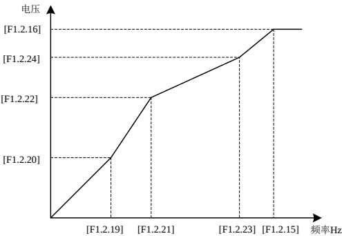
图 7-28 V/F 自定义曲线
