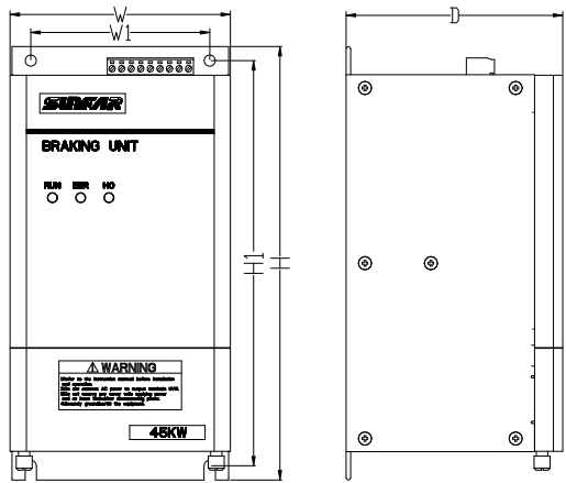
图 12-3 安装尺寸图
