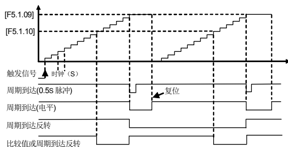
图 7-41-B 定时器 1 周期达到基本功能示意图 (F5.1.06=10#1)
