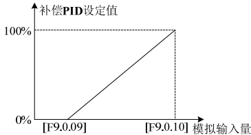
图 7-65 补偿 PID 设定值定义示意图
