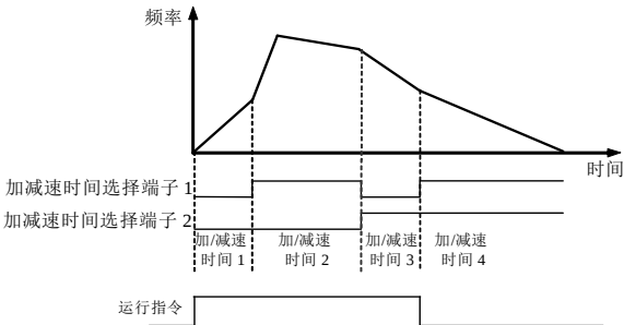
图 7-25 加、减速时间的外部端子选择方式
