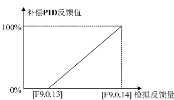
图 7-66 补偿 PID 反馈值定义示意图
