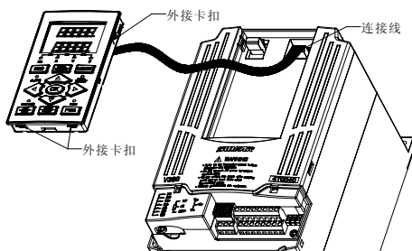
图 3-7 外延键盘连线图
