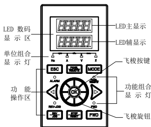
图 3-4-B 双 LED 飞梭型
