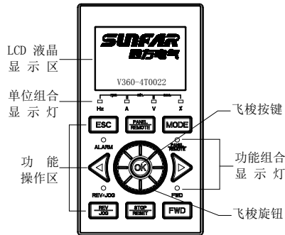
图 12-7-B 双语 LCD 飞梭型 (型号 DPNL360CB /PN: 050M007360002)
