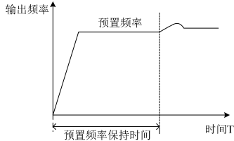
图 7-57 闭环预置频率运行示意图
