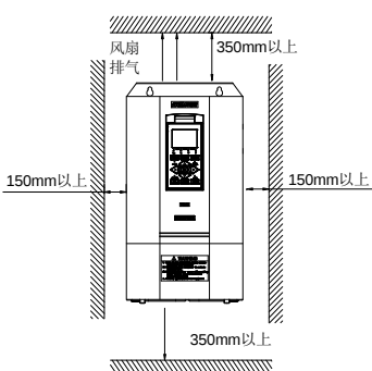
图 3-1-B 安装的间隔距离(45KW 以上)
