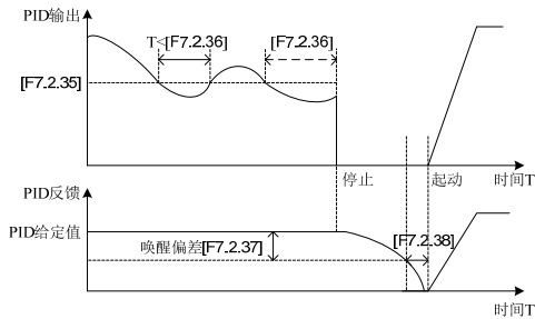
图 7-59 PID 睡眠功能示意图
