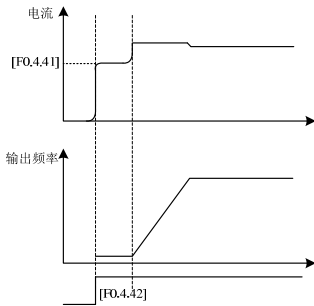
图 7-18 起动预励磁输出
