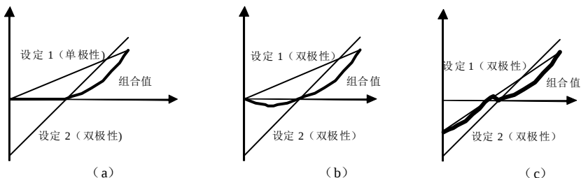
图 7-9-E 频率组合示意图 5
