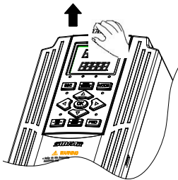
图 3-5 操作面板拆卸示意图
