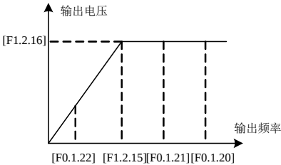
图 7-10 频率参数定义示意图
