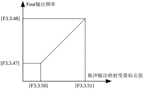
图 7-35 脉冲输出 Fout 特性曲线
