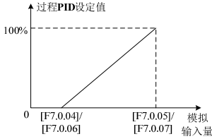
图 7-52 过程 PID 设定值定义示意图
