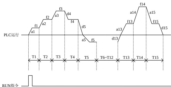
图 7-48-B 简易 PLC 运行单循环模式
