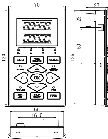
图 3-10-A 操作面板安装尺寸 1
