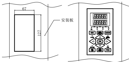
图 3-10-C 操作面板安装尺寸 3
