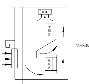
图 3-2 两台变频器上下安装间隔
