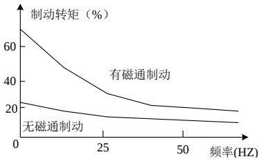
图 7-43 磁通制动曲线
