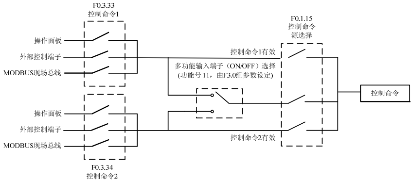
图 7-7 控制命令源选择示意图
