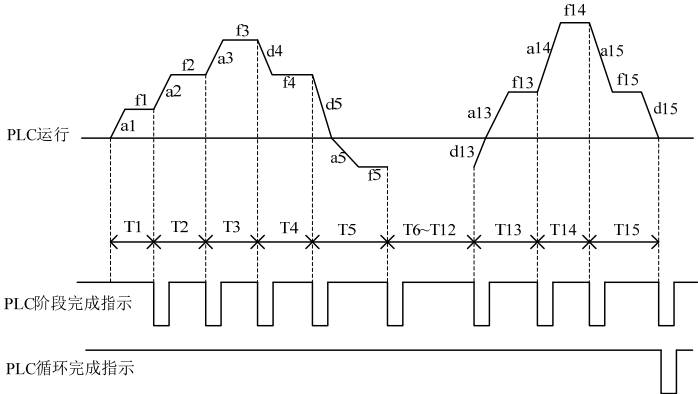
图 7-48-A 简易 PLC 运行
