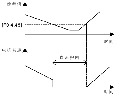
图 7-19 直流抱闸示意图
