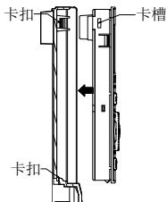
图 3-6 操作面板安装示意图
