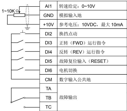
图 7-4 机床主轴驱动宏 AI1 设定接线图
