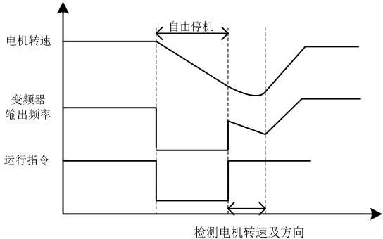
图 7-16 转速跟踪启动示意图
