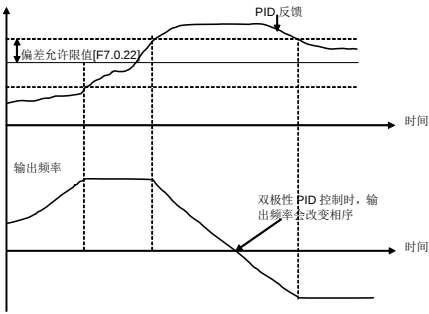
图 7-55-B 双极性 PID 控制方式
