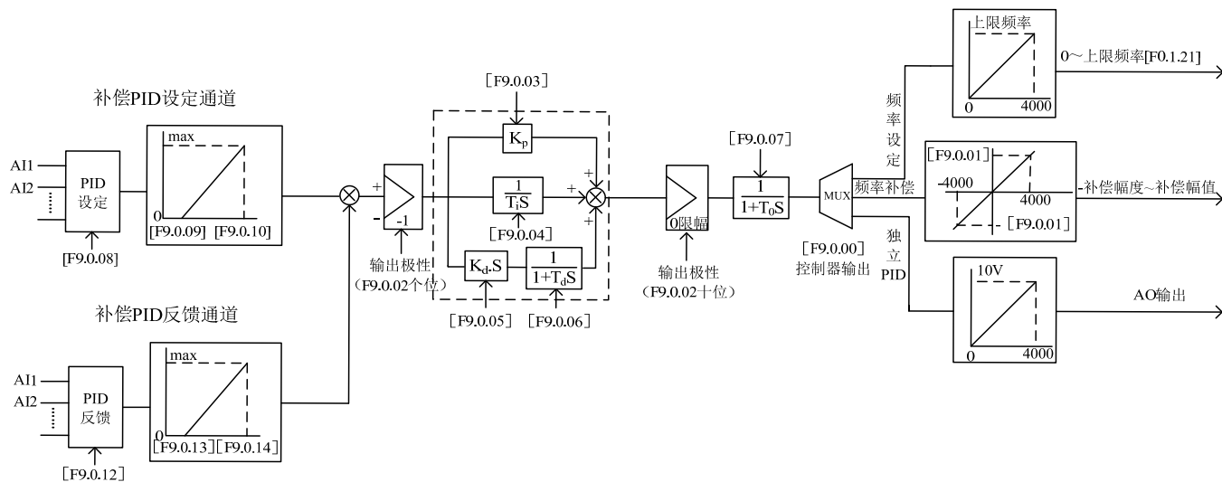
图 7-64 补偿 PID 原理框图
