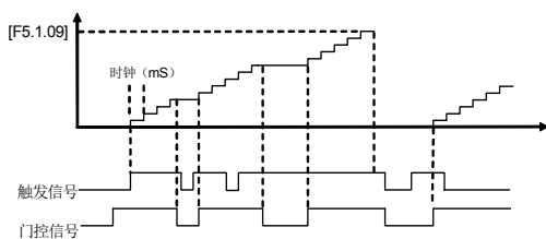
图 7-41-C 定时器 1 (UT1) 的起动触发、门控信号功能 (F5.1.06=1111; F5.1.15=0001)
