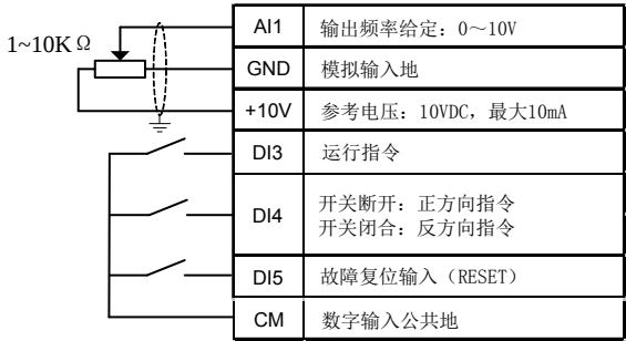
图 7-2-B 两线控制二 AI1 设定接线图
