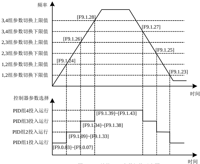
图 7-67 补偿 PID 参数切换示意图
