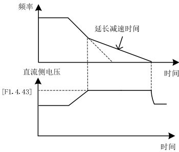
图 7-31-B 减速过程的过压抑制
