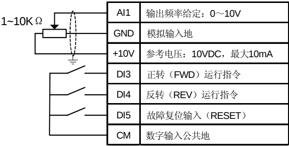
图 7-2-A 两线控制一 AI1 设定接线图
