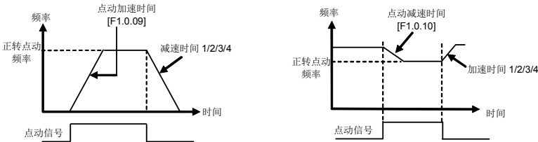
图 7-11 正转点动运行曲线
