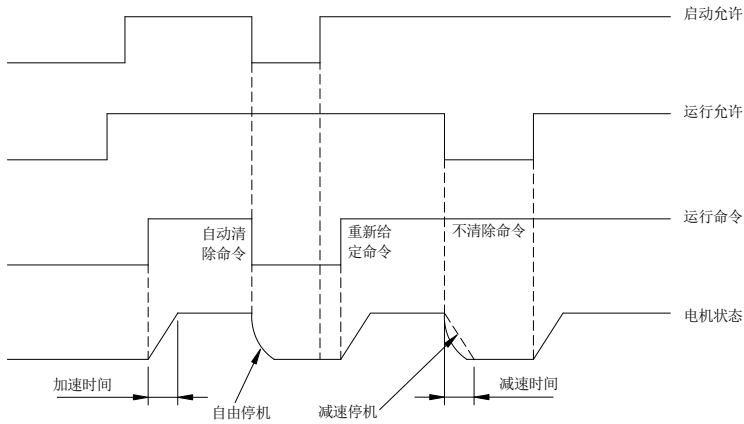
图 7-15 启动过程原理图
