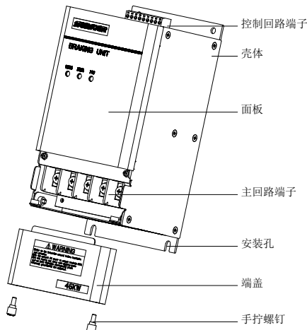
图 12-2 外观示意图
