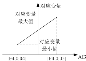
图 7-37-A AI3 模拟输入与对应变量示意图(单极性)
