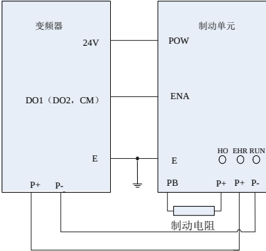
图 12-4 接线示意图
