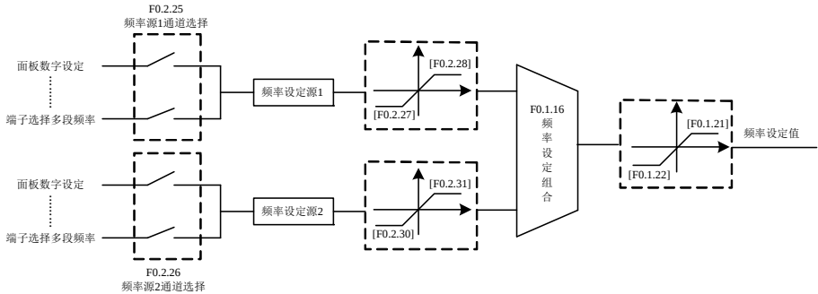
图 7-8 频率设定通道结构示意图
