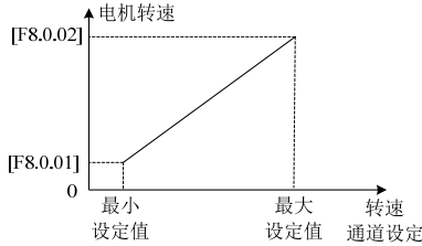
图 7-61 转速设定值和电机转速对应关系图
