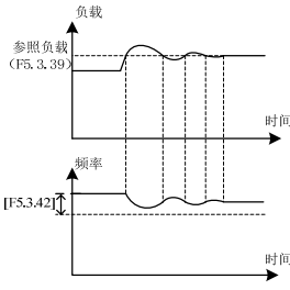
图 7-45 负载动平衡功能示意图
