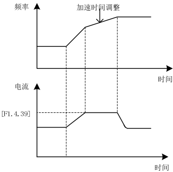
图 7-30 加/减速电流限制示意
