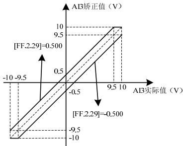
图 7-71-A AI3 零偏矫正曲线
