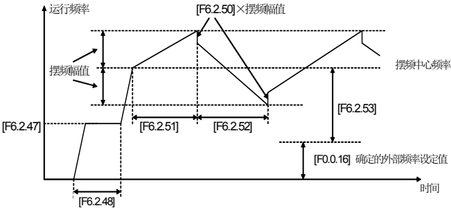
图 7-50 摆频运行示意图
