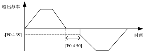
图 7-22 起动频率正反切换示意图
