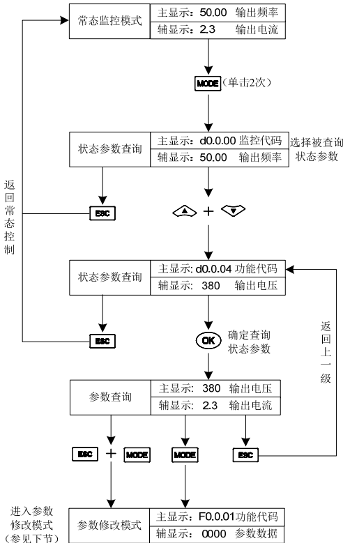
图 5-1 状态参数查询示意图
