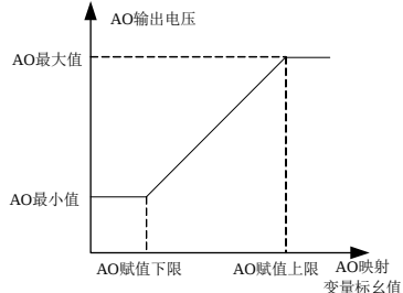
图 7-39 AO 输出特性曲线
