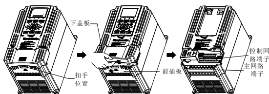
图 3-4 塑壳盖板的拆卸安装示意图
