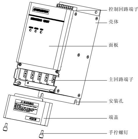
图 13-2 外观示意图
