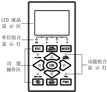
图 13-7-A 双语 LCD 标准型 (型号 DPNL360CA /PN: 050M007360001)
