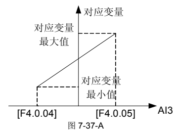
AI3 模拟输入与对应变量示意图(单极性)
