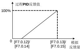
图 7-53 过程 PID 反馈值对应关系示意图
