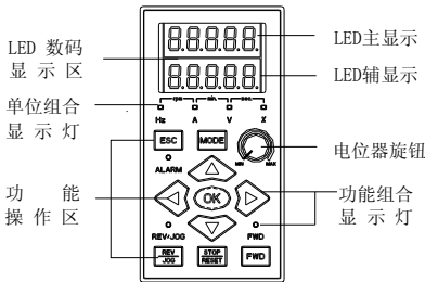
图 13-7-C 双行 LED 电位器小面板 (型号 DPNL350EN /PN: 050M007033601)
