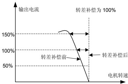
图 7-29 转差频率补偿示意图
