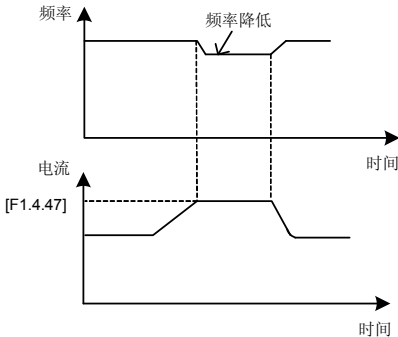
图 7-32-B 限流调节示意图
