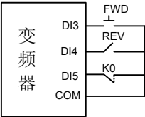
图 7-14-B 三线式运行模式 2
