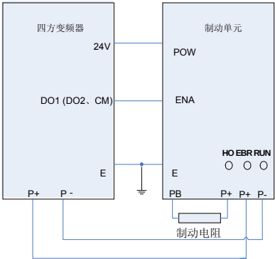
图 13-4 接线示意图
