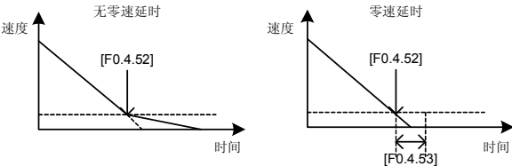
图 7-23 有无零速延时对比图
