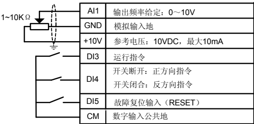
图 7-2-A 两线控制一 AI1 设定接线
