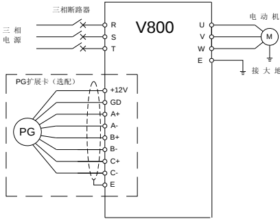
图 5-4 VC 模式运行接线
