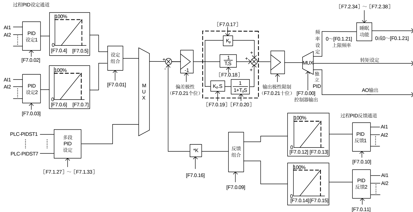
图 7-51 过程 PID 控制原理框图
