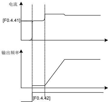
图 7-18 启动预励磁输出
