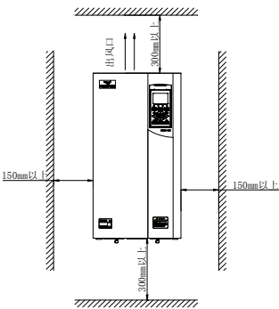
图 3-1-B 安装的间隔距离(37KW 及以上)
