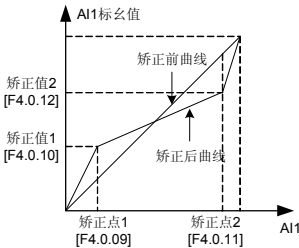
图 7-38 模拟输入 AI1 曲线
