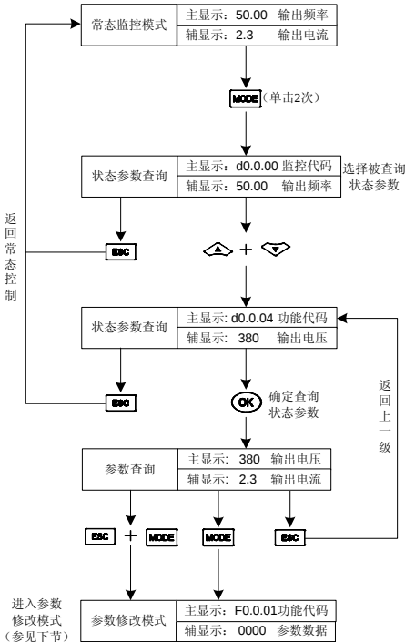
图 5-1 状态参数查询示意图
