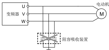
图 4-1 输出端禁止连接阻容吸收装置
