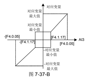
AI3 模拟输入与对应变量示意图(双极性)
