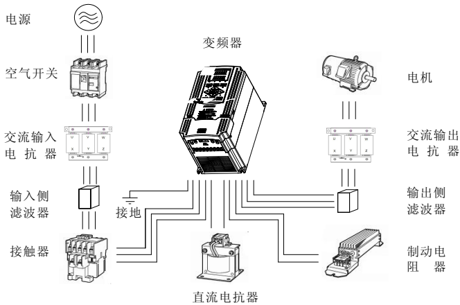
图 4-2 变频器的配线
