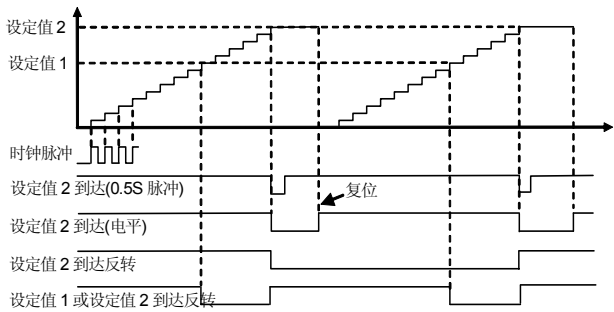
图 7-42-B 计数器功能 2
