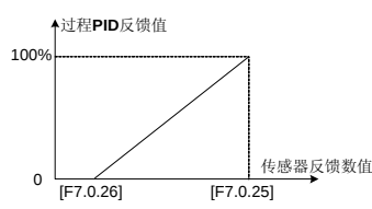
图 7-58 反馈百分比与对应传感器数值的对应关系曲线
