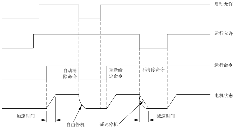
图 7-15 启动过程原理图
