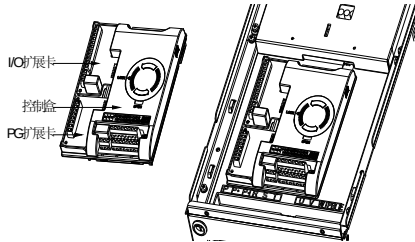
图 3-6 扩展卡的拆卸安装示意图
