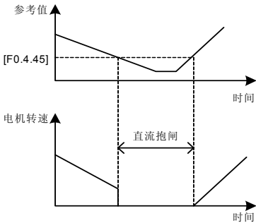
图 7-19 直流抱闸示意图
