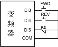
图 7-14-A 三线式运行模式 1
