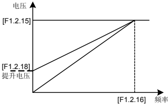
图 7-27-B 恒转矩曲线转矩提升示意图
