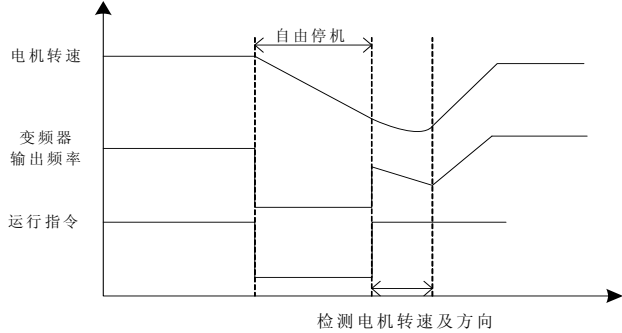
图 7-16 转速跟踪启动示意图
