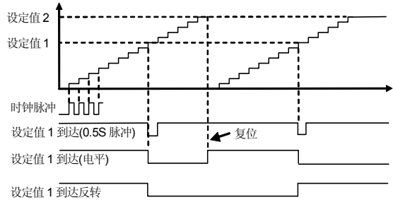
图 7-42-A 计数器功能 1
