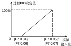
图 7-52 过程 PID 设定值定义示意图
