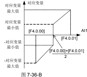
AI1 模拟输入与对应变量示意图(双极性)
