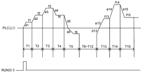
图 7-48-E 简易 PLC 运行保持最终值模式
