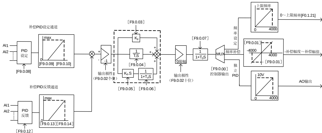
图 7-64 补偿 PID 原理框图
