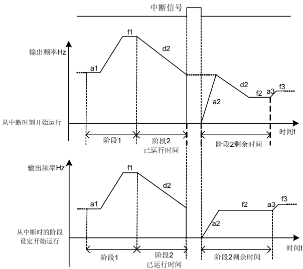
图 7-49 断点恢复示意图
