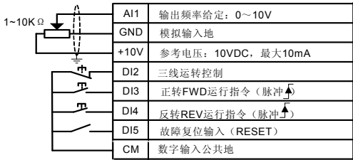
图 7-3 三线控制一/AI1 设定接线图
