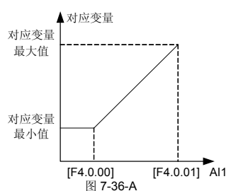
AI1 模拟输入与对应变量示意图 (单极性)
