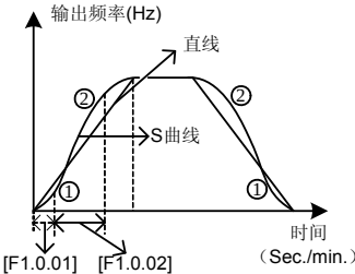
图 7-24 加减速曲线
