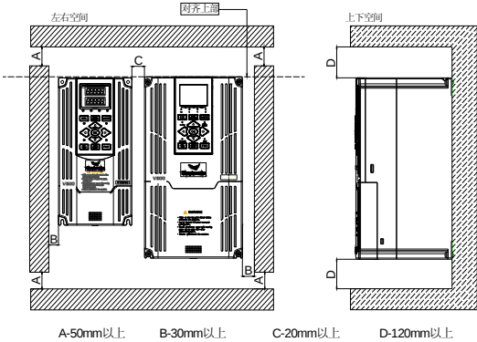
图 3-3 两台变频器（4.0KW 以上）左右安装尺寸
