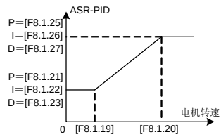
图 7-63-B 双 PID 参数（连续切换）
