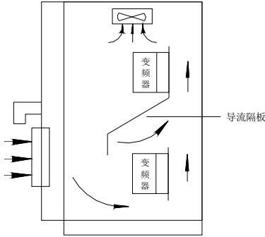
图 3-2 两台变频器上下安装间隔
