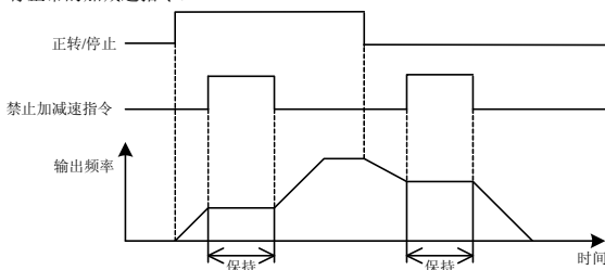
图 7-33 禁止加减速示意图
