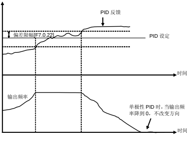
图 7-55-A 单极性 PID 控制方式
