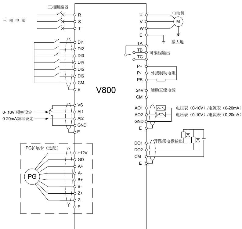
图 4-3 V800 系列变频器基本接线图
