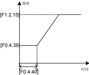
图 7-17 起动频率示意图
