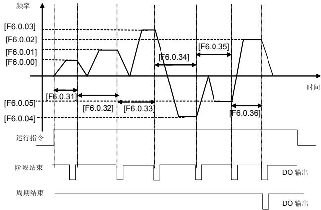
图 7-48-C 简易 PLC 运行单循环停机模式
