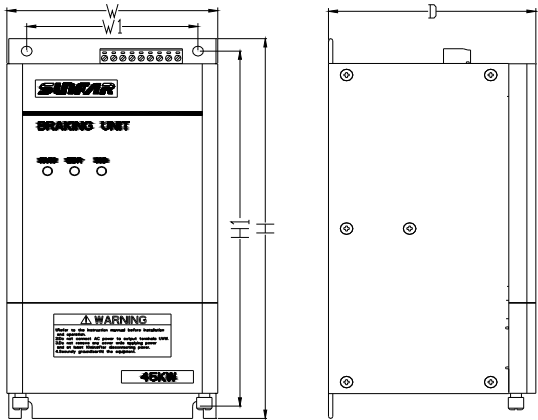
图 13-3 安装尺寸图
