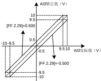
图 7-71-A AI3 零偏矫正曲线
