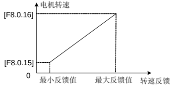
图 7-62 转速反馈值和电机转速对应关系图
