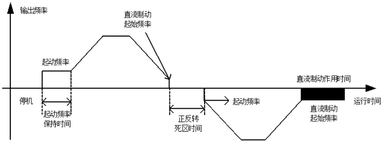
图 7-20 停机直流制动示意图
