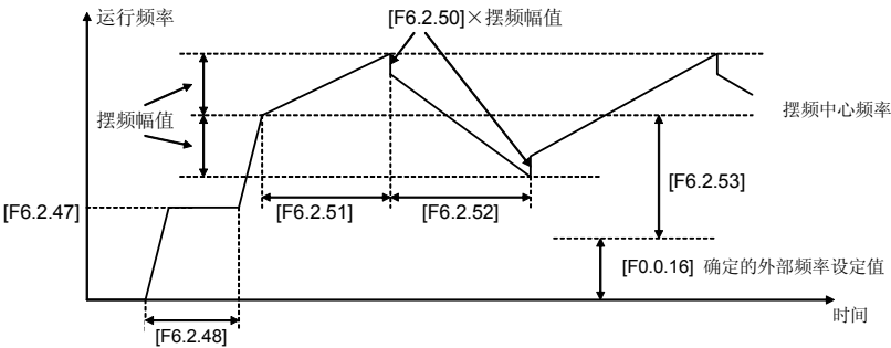
图 7-50 摆频运行示意图
