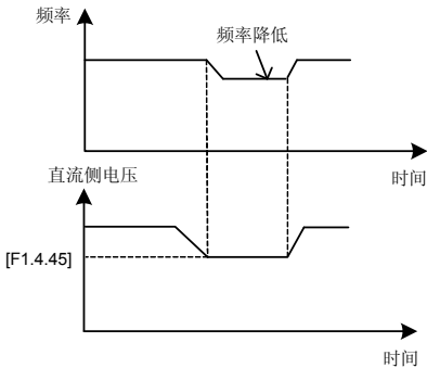
图 7-32-A 欠压调节示意图
