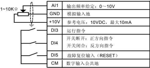
图 7-2-B 两线控制二 AI1 设定接线图
