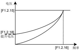
图 7-27-A 降转矩曲线转矩提升示意图
