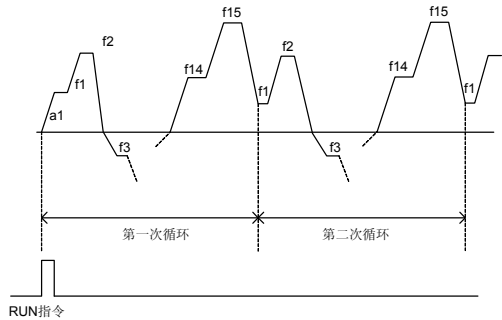
图 7-48-D 简易 PLC 运行连续循环模式
