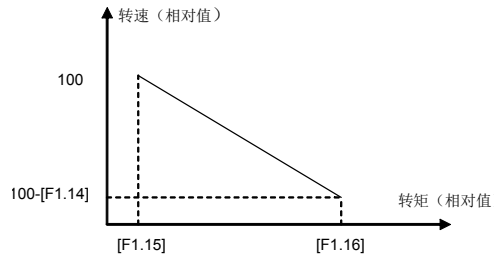
图 6-9 下垂控制作用时的电机特性
