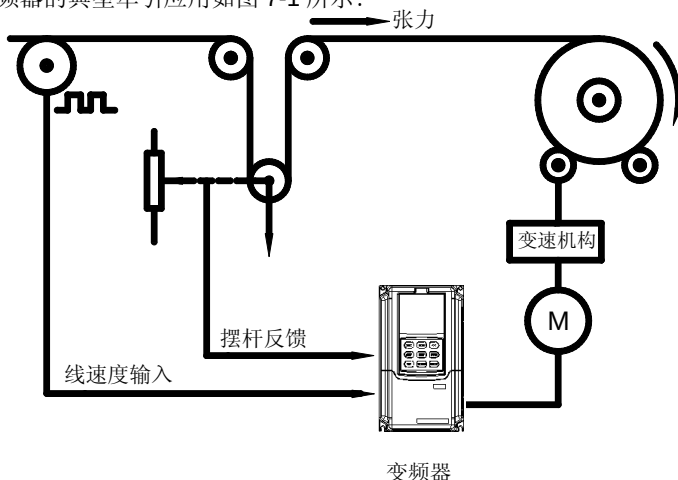
图 7-1 典型牵引应用
