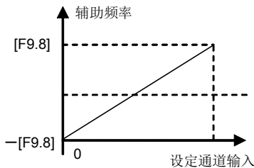
图 6-34 辅助频率的调整幅度
