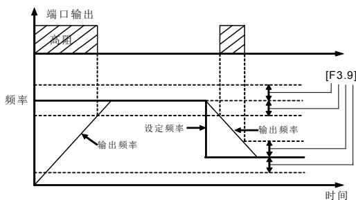
图 6-14 频率到达信号
