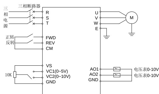
图 10-2 基本接线图
