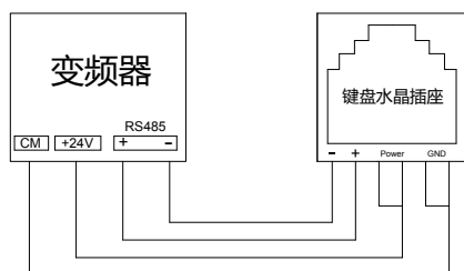
图 B-6 接线方式 1
