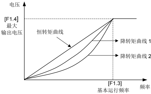
图 6-4 V/F 曲线
