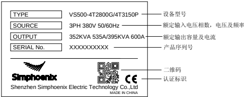
图-1 变频器铭牌数据
