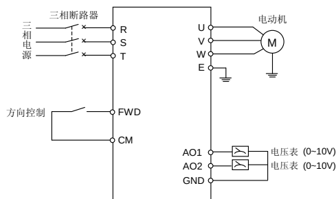
图 10-1 基本接线
