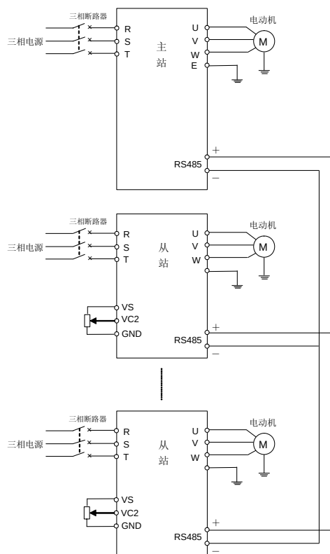
图 10-4 基本接线图
