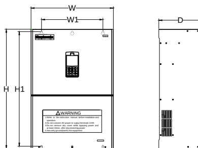
图 2-4-C 变频器的安装尺寸
