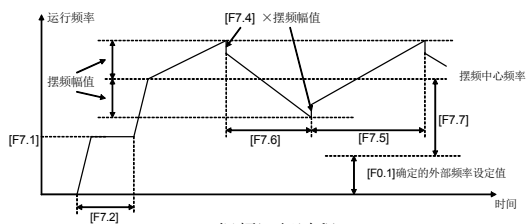
6-27 摆频运行过程
