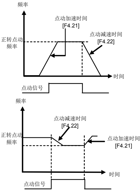
图 6-19 点动运行
