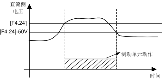
图 6-23 能耗制动
