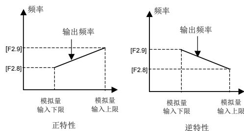
图6-10 模拟输入与设定频率对应图
