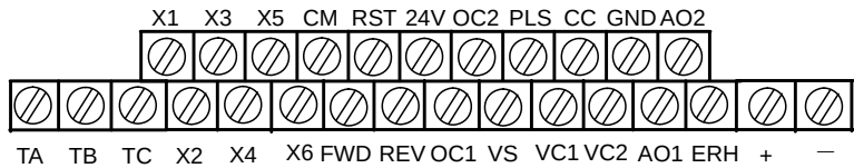
图 3-4 控制回路端子示意图
