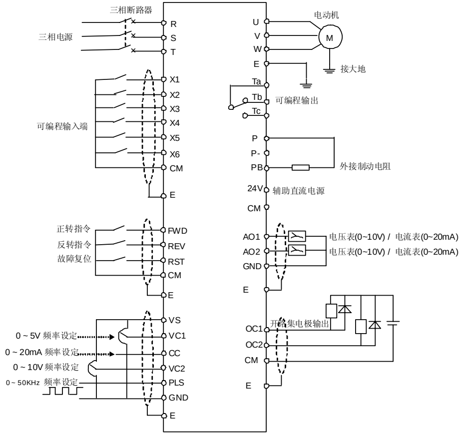
图 3-3 VS500 系列变频器基本接线图
