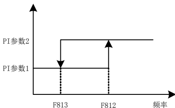
图 6-22 增益切换示意图
