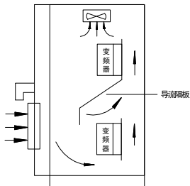
图 2-1-C 多台变频器的安装
