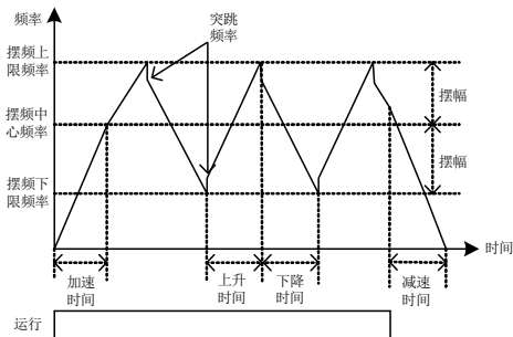
图 6-19 摆频运行示意图
