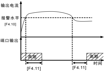
图 6-17 过载报警
