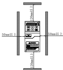
图 2-1-B 安装的间隔距离
