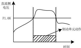
图 6-7 能耗制动
